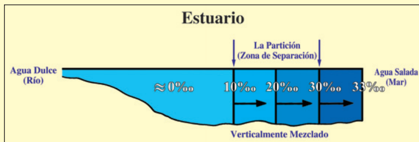
Figura 14: Corte longitudinal que muestra la salinidad (partes por mil 0/00), en un estuario. Aquí podemos observar la partición (Zona de separación), entre el agua dulce y la salada. (Levemente modificado de Introductory Oceanography [Oceanografía Introductoria], Thurman, p. 301.)
