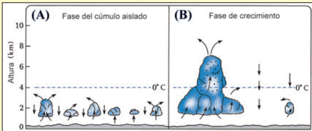
Figura 19: (A) Pequeños pedazos sueltos de nubes (cúmulos). (B) Cuando las pequeñas nubes se juntan las corrientes de aire en la gran nube aumentan, haciendo que la nube vaya tomando la forma de una pila. Las gotas de agua están indicadas con (.). ( The Atmosphere [La Atmósfera], Anthes y otros, p. 269.)
