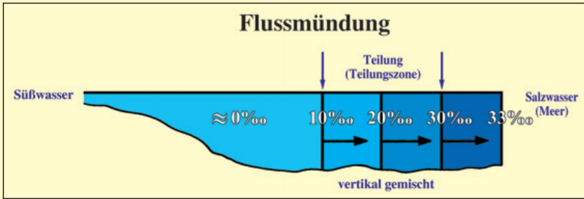
Abbildung 14: Längsschnitt, der den Salzgehalt (Parts per million ‰) an einer Mündung zeigt. Wir können hier die Aufteilung zwischen frischem und salzigem Wasser sehen (Separationszone). ( Oceanography [Ozeanographie], Thurman, S.301, mit einer leichten Verbesserung.)
